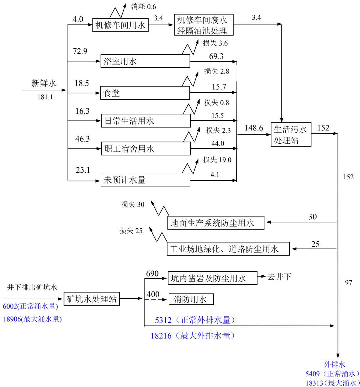
图 2—13 矿山开采给排水平衡图 (单位: m 3 /d)
